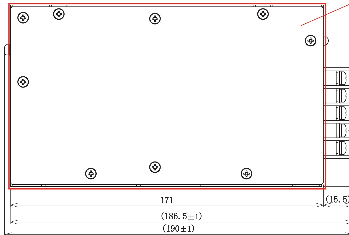
底面図
