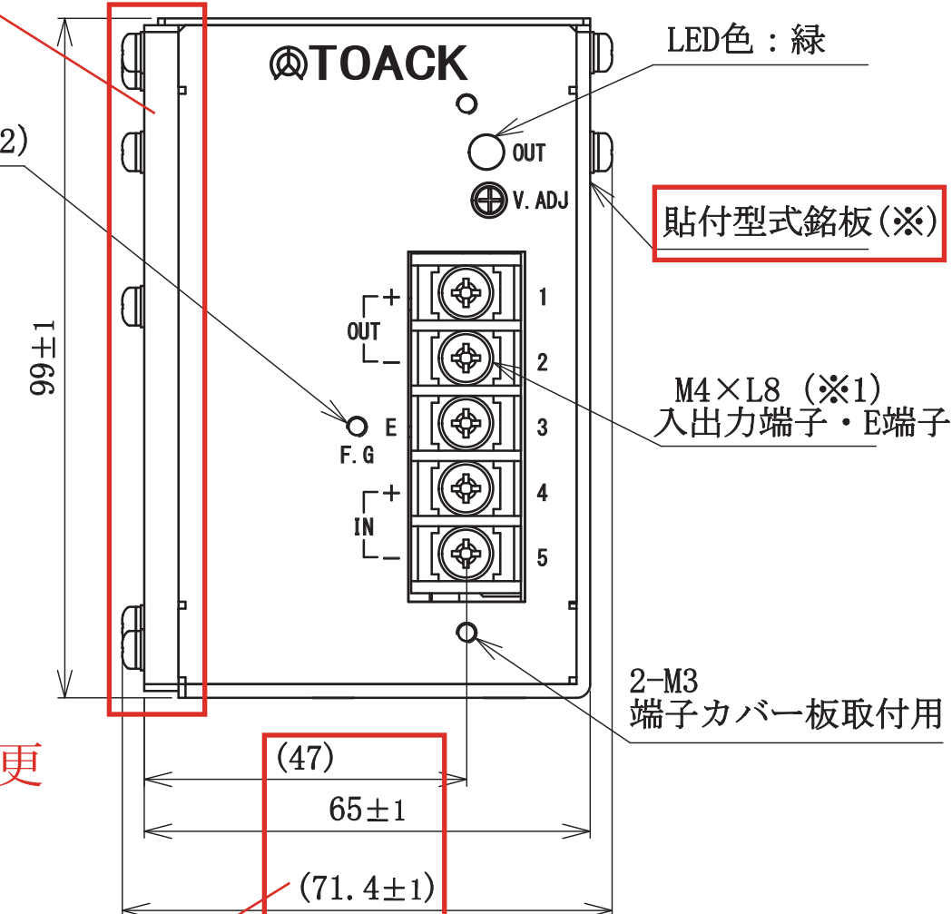
正面図
